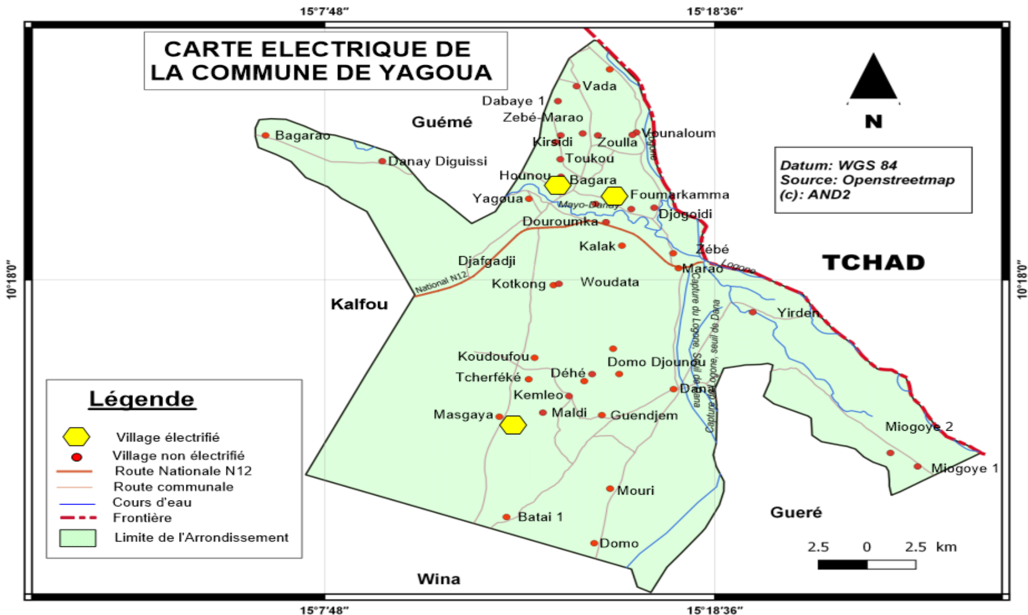
Carte 5 : Infrastructures électriques
